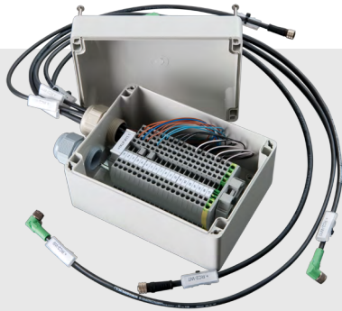
组装标准机箱
